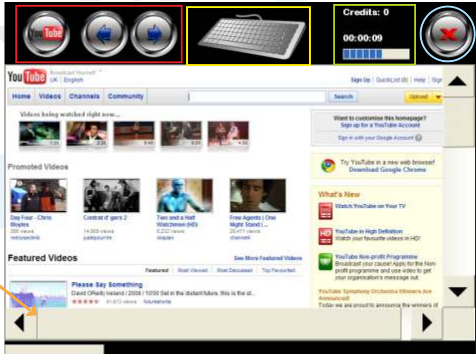
fig. 1.6.1 - YouTube screen
